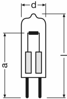
HALOSTAR 24 V 20 W 24 V G4
