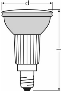
HALOPAR 16 ST 40 W 230 V 35° E14
